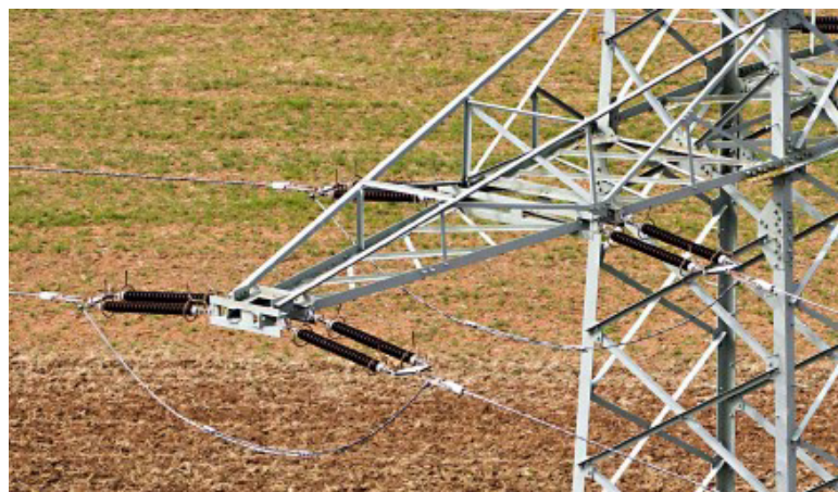
Abbildung 6: Abspannkette
